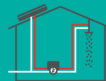
Le SUNPAD est connecté en série avec un chauffe-eau instantané
