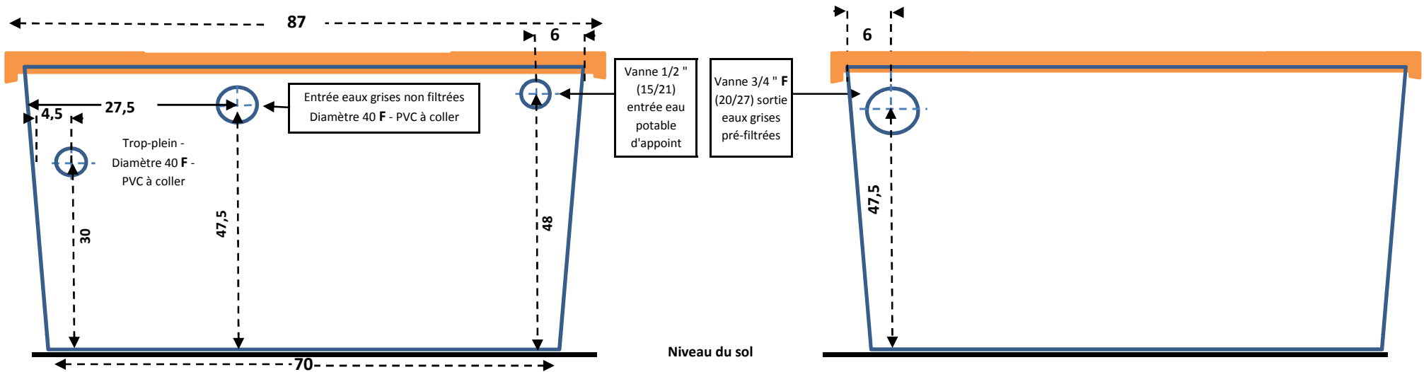
Face 1 - entrée des eaux grises dans SPAREAU
